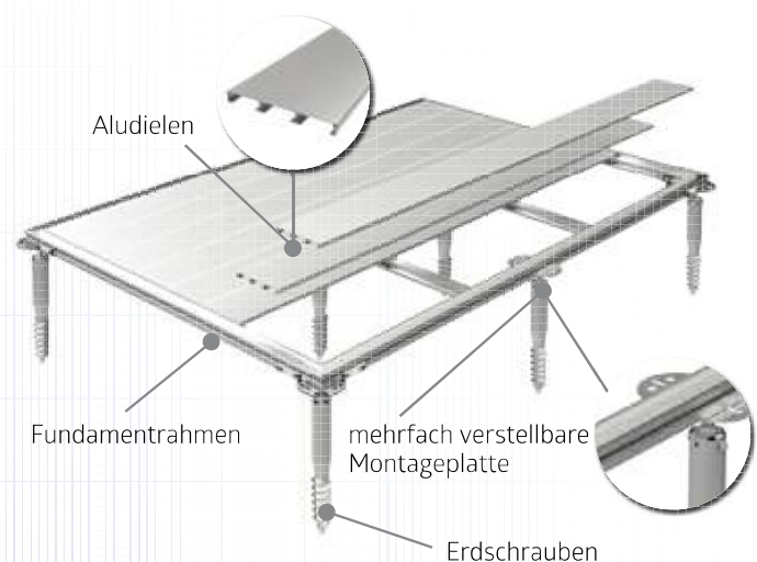
Abb. Erdschrauben-Fundament
